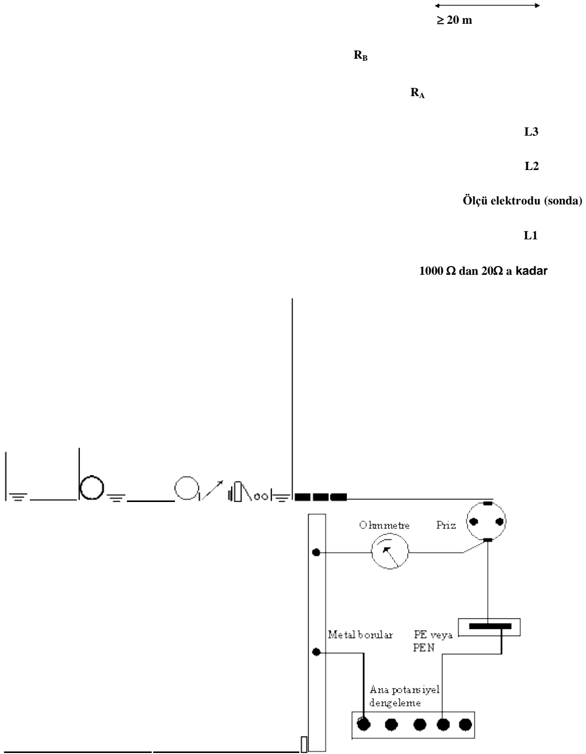
Şekil-8a Koruma iletkenlerinin bağlantısının ölçülmesi Şekil-8b Topraklama direncinin ölçülmesi için örnek
