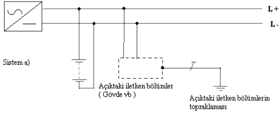
Şekil-5j TT Doğru akım sistemi
