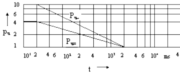
Şekil-Y.8 Etki süresine t bağlı olarak kısa süre katsayıları p_{r-} ve p_{r+} 'nin değişimi
