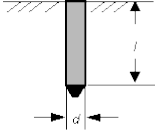
Şekil-T.6 Derin (çubuk) topraklayıcı
